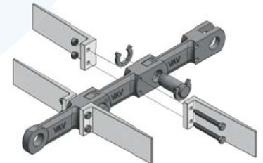
Einfach anzubringende/abnehmbare Kunststoffschaber
