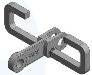
„O“-Form für vertikaler Transport
