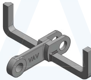
„U“-Form für geneigter Transport
